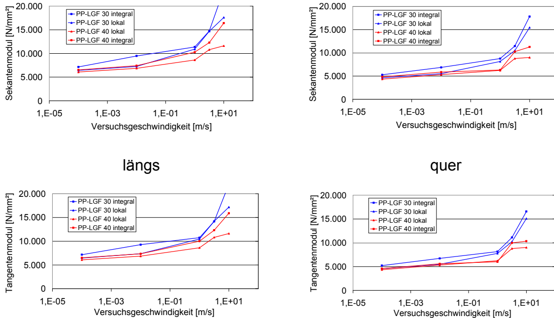
Abb. 7.1: Veränderung der Anfangssteifigkeit bei zunehmender Abzugsgeschwindigkeit, , Faserorientierung in Zugrichtung (links), Faserorientierung quer zur Zugrichtung (rechts), Auswertung nach DIN (oben), Berechnung der Tangente bei 0,15% Dehnung (unten)
