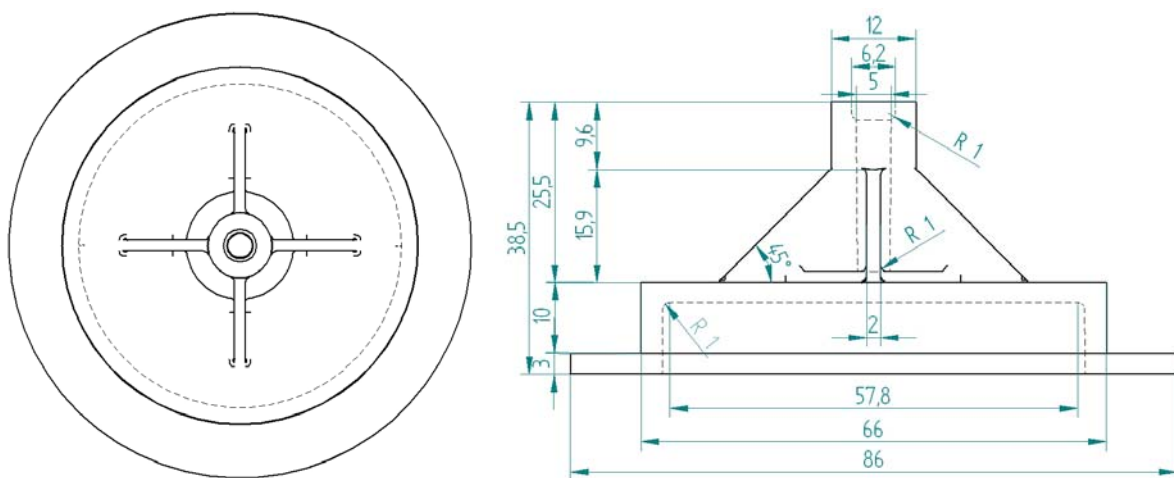
Abb. 3.17: Befestigungsdemonstrator mit 45°-Rippen
