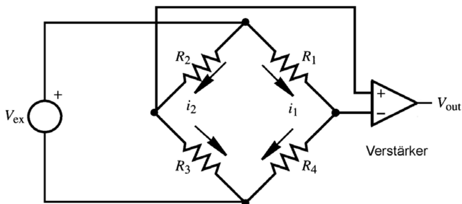
Abb. 4.7: Schaltkreis der dynamischen Wheatstoneschen Brückenschaltung [110].
