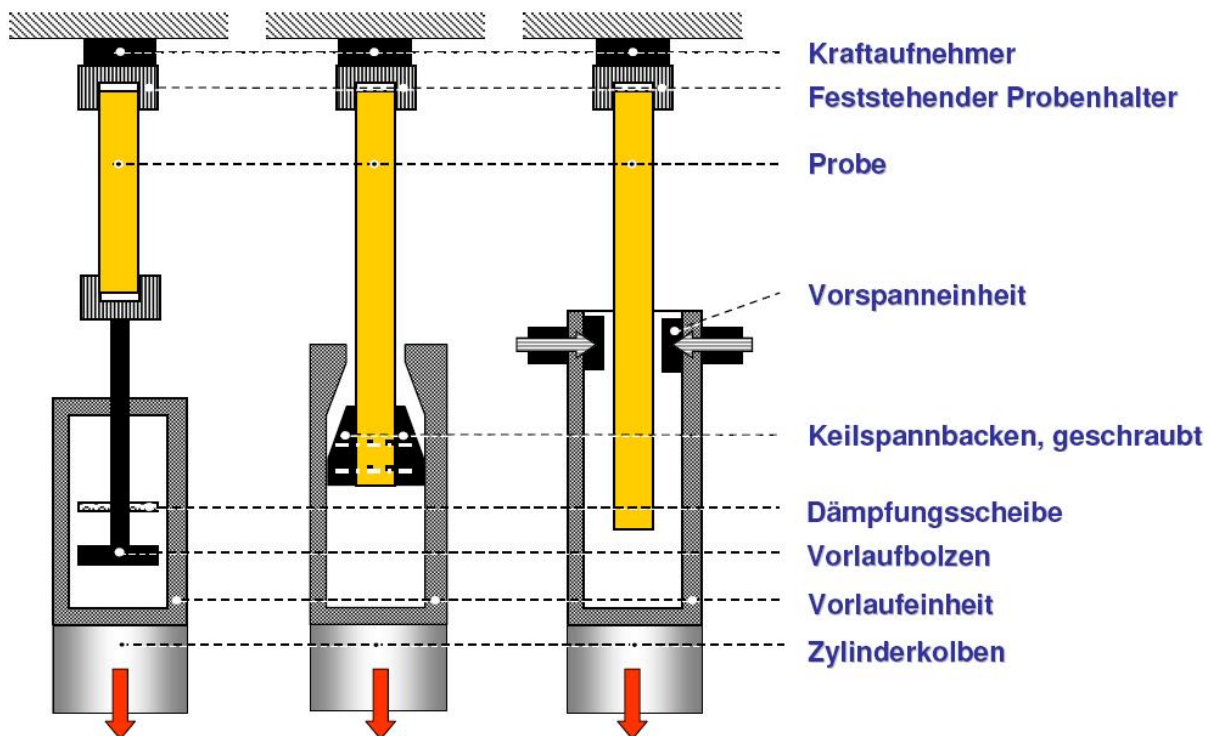
Abb. 4.4: Spannvorrichtung für Hochgeschwindigkeitszugversuche [105]
