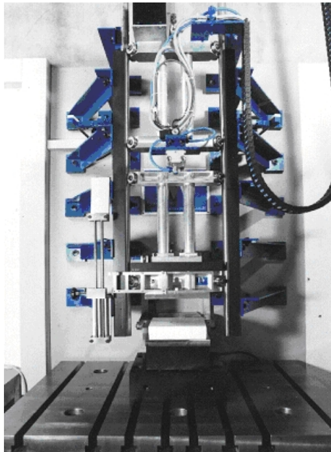
Abb. 4.2: Fallgewichtsanlage [101]
