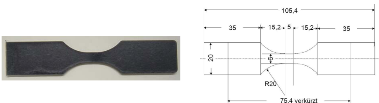
Abb. 3.7: Abmessungen der Zugprobe, Probekörper (links), Skizze (rechts)
