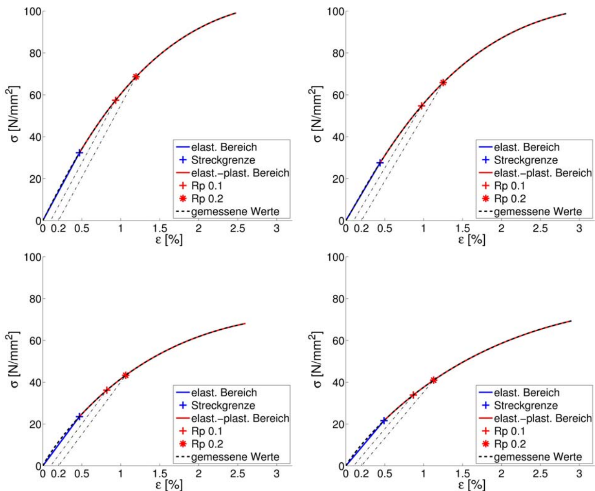
Abb. 7.25: Elastischer und plastischer Bereich der Spannungs-Dehnungs-Beziehung, Darstellung der Streckgrenze und der Ersatzstreckgrenzen R_p 0,1 und R_p 0,2 , PP-LGF 30, Faserorientierung in Belastungsrichtung (oben) und quer dazu (unten), integrale Auswertung (links), lokale Auswertung (rechts)
