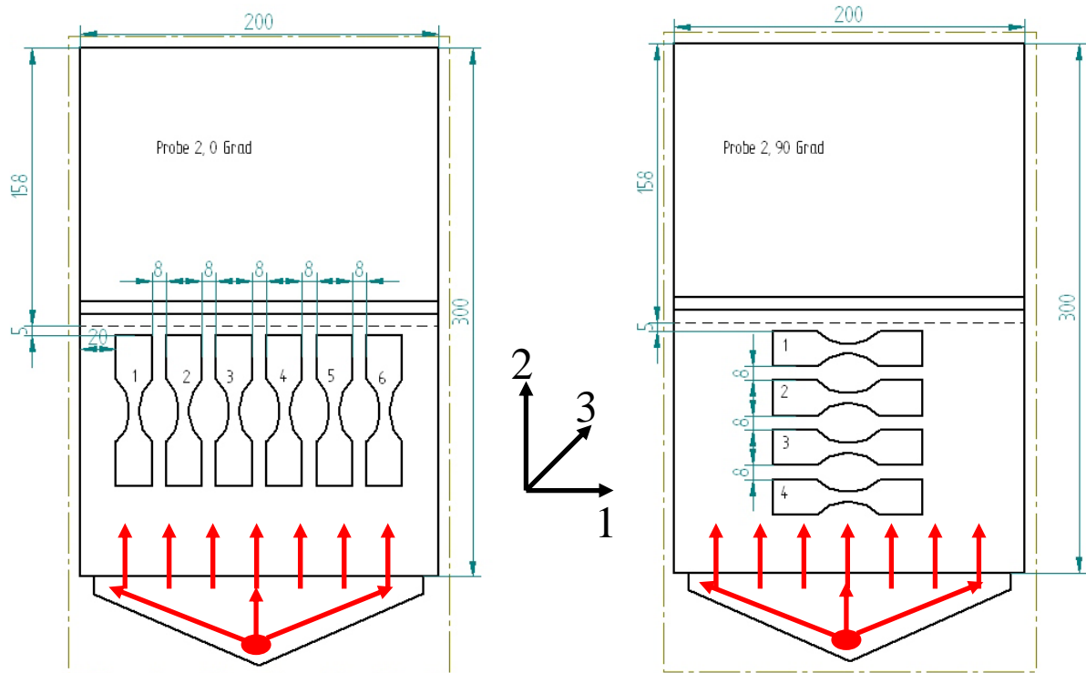
Abb. 3.12: Entnahmeplan für Zugproben (PP-LGF 40 Celstran) in Faserlängsrichtung (links) und quer (rechts), Daimler-Platte
