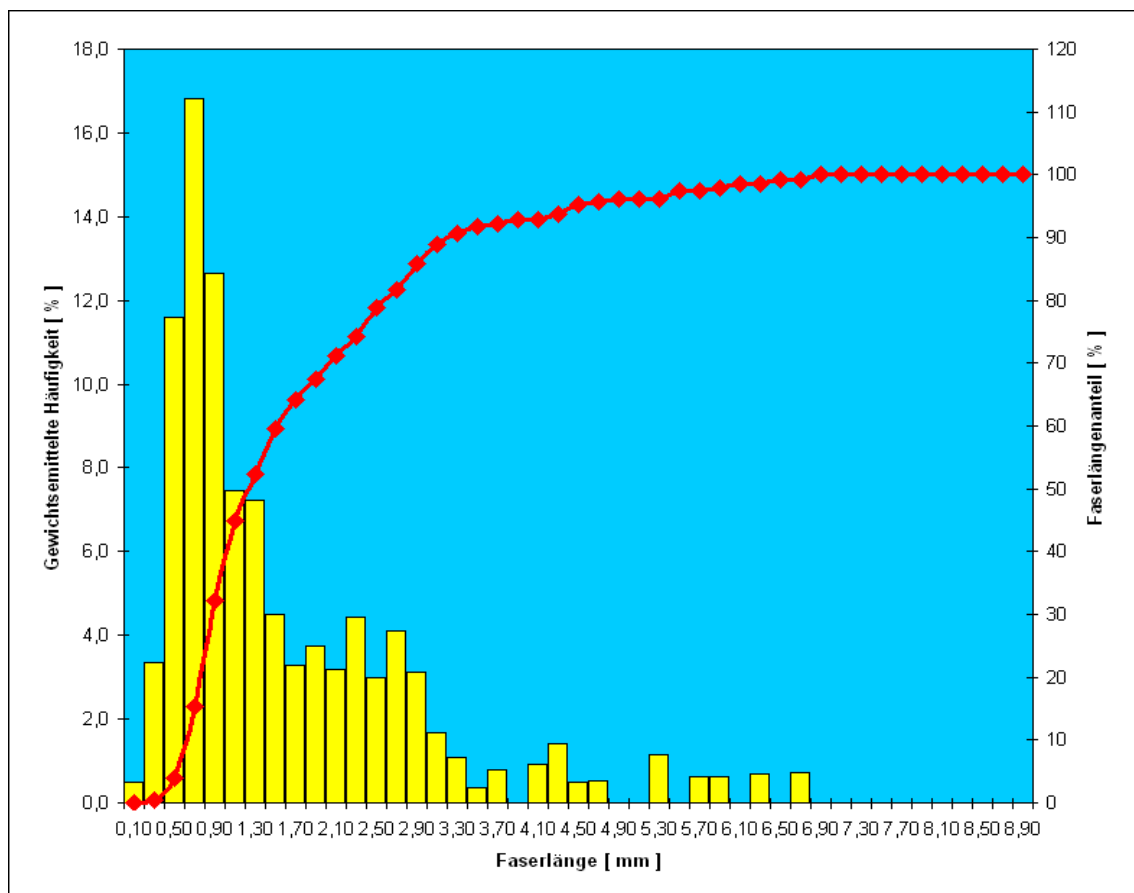
Abb. 5.14: Gewichtsgemittelte Häufigkeit der Faserlängen, Probekörper aus PP-LGF 30
