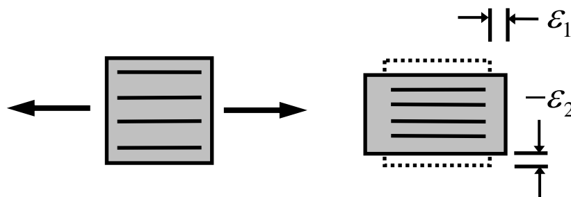
Abb. 2.2: Dehnungs-Querdehnungskopplung
