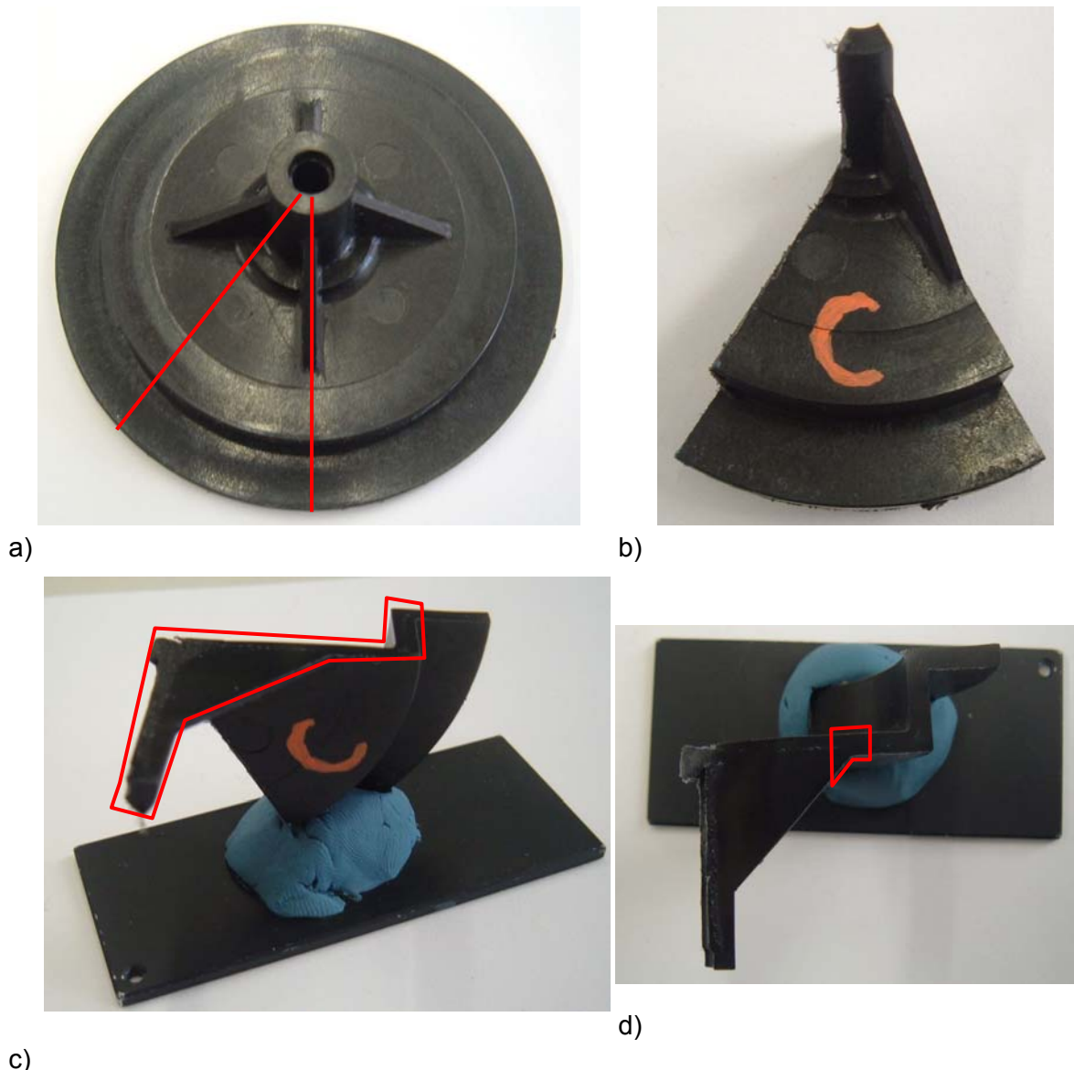
Abb. 5.38: Vorbereitungen für und Lage der Schliiffbilder an Bauteildemonstrator mit 45°-Rippen: a) Schnittkanten, b) heraus geschnittenes Teilstück, c) präparierter Bereich, d) Übergang der Rippe in flachen Teil (Bereich für Detailaufnahme)
