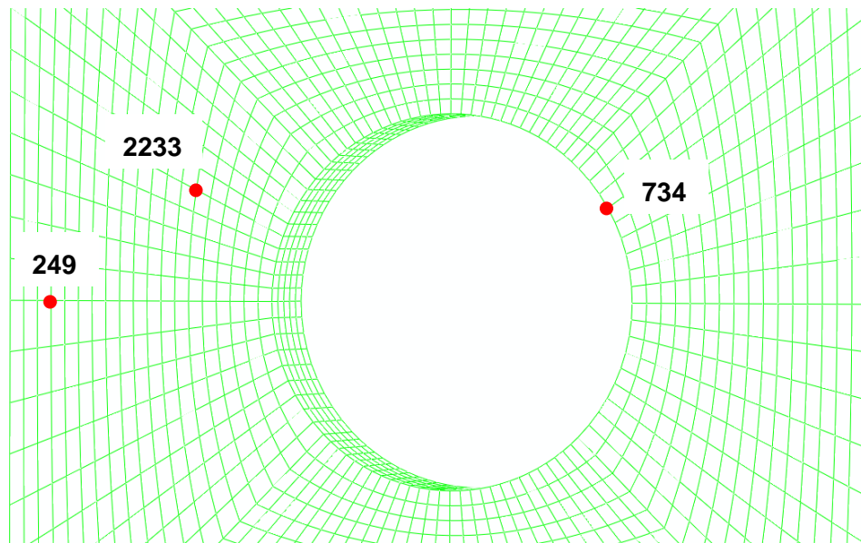
Abb. 8.10: Lage der FE-Knoten für die Validierung
