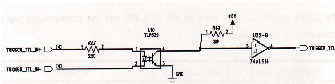
Abb. 4.11: Schaltplan für den internen Signallaufweg des Triggersignals in der HG-Kamera Fehler!
