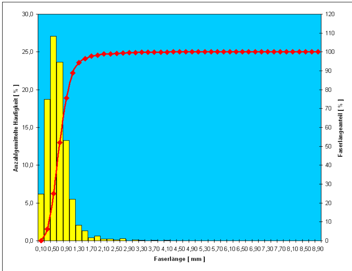
Abb. 5.13: Anzahlgemittelte Häufigkeit der Faserlängen, Probekörper aus PP-LGF 40
