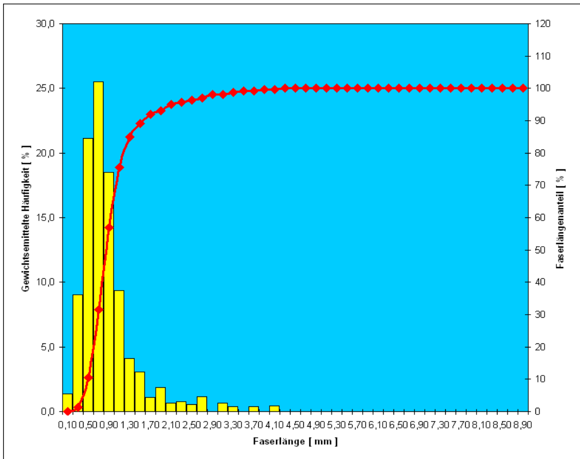
Abb. 5.15: Gewichtsmittelte Häufigkeit der Faserlängen, Probekörper aus PP-LGF 40 Eine weitere Kenngröße ist die mittlere Faserlänge. Sie ergibt sich zu:
