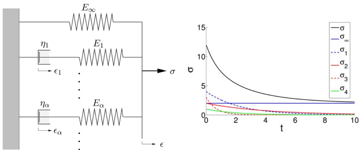
Abb. 2.8: verallgemeinertes Maxwell-Modell, Spannungsverlauf im Relaxationsversuch und Spannungsanteile der einzelnen Elemente (n=5)
