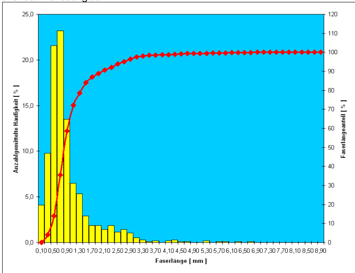
Abb. 5.12: Anzahlgemittelte Häufigkeit der Faserlängen, Probekörper aus PP-LGF 30
