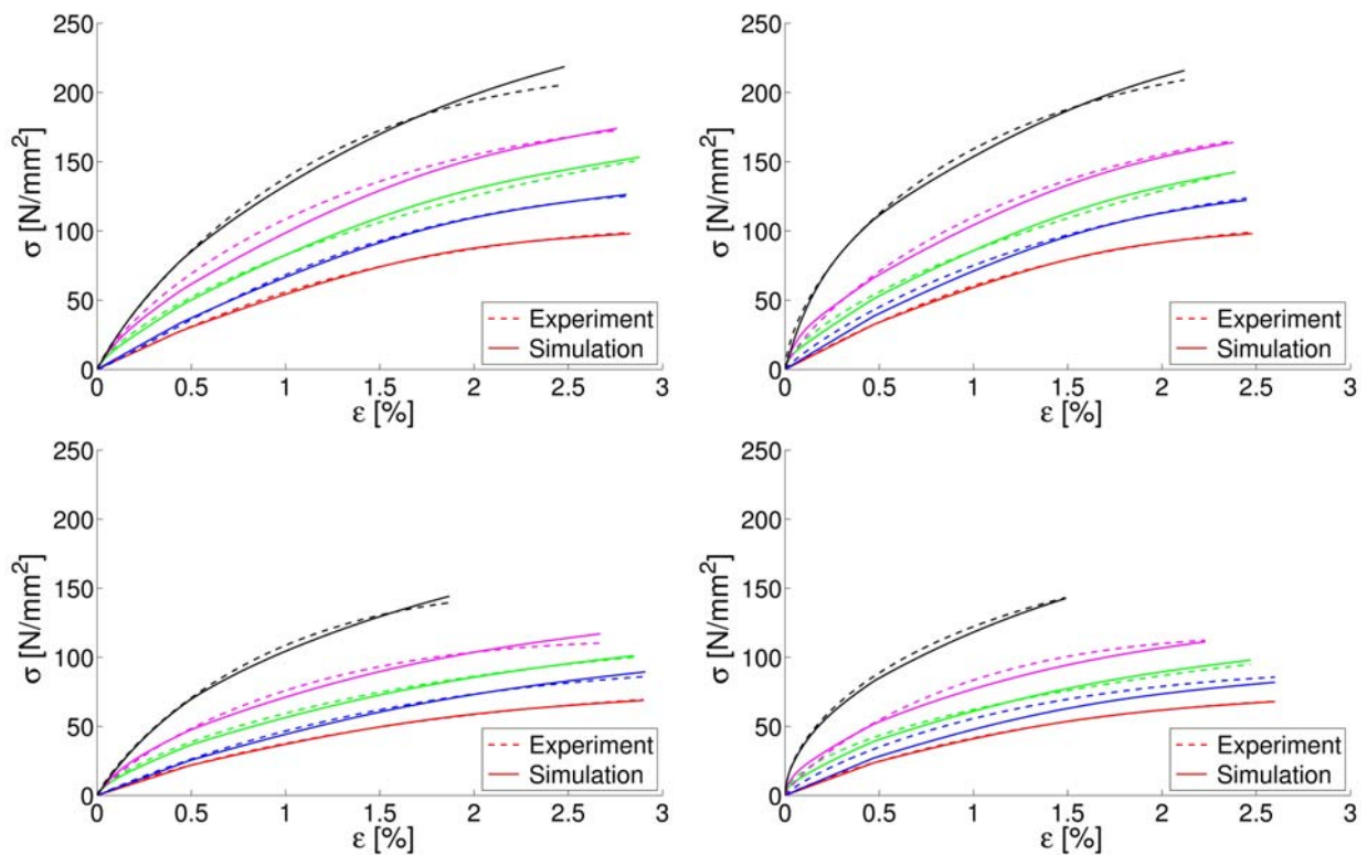
Abb. 7.29: Vergleich gemessener und simulierter Dehnratenspektren, PP-LGF 30, Fasern in Zugrichtung (oben), Fasern quer zur Zugrichtung (unten), lokale Auswertung am Versagensort (links), gemittelte Dehnung in Probenmitte (rechts)
