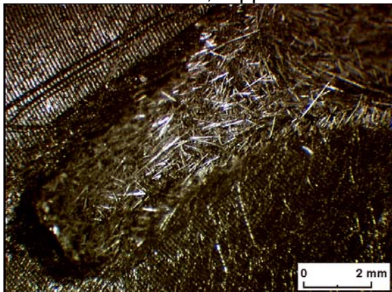
PP-LGF 30, Rippenendbereich
