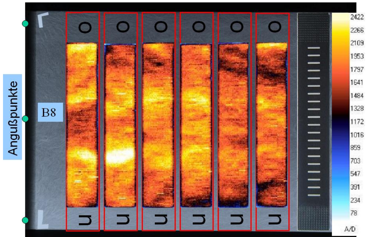
Abb. 5.4: Untersuchung der Homogenität einer Probestabplatte aus PP-LGF 30 mit der TSA, Querorientierung der Fasern innerhalb der Probestäbe
