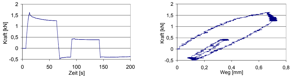
Abb. 7.23: Kraft-Zeit-Verläufe (links) und Kraft-Weg-Verläufe (rechts) für Versuchsart 1 (oben) und Versuchsart 2 (unten), Fasern parallel zur Zugrichtung
