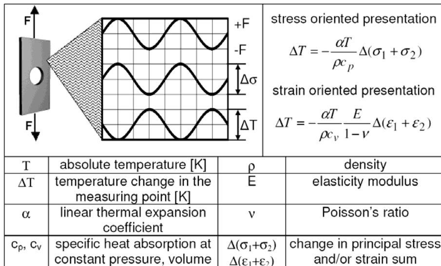
Abb. 5.1: Thermoelastischer Effekt [137]
