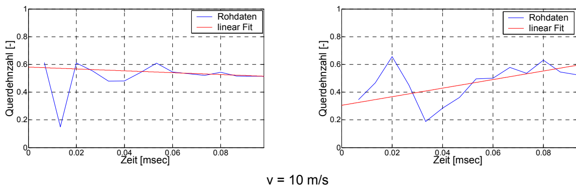
Abb. 7.7: Zeitlicher Verlauf der Querdehnzahl bei hohen Abzugsgeschwindigkeiten, PP-LGF 40, Zugversuche quer zur Faserrichtung, Betrachtung der Schmalseite der Probe, links: flächige Auswertung in Probekörpermitte, rechts: lokale Auswertung am Versagensort
