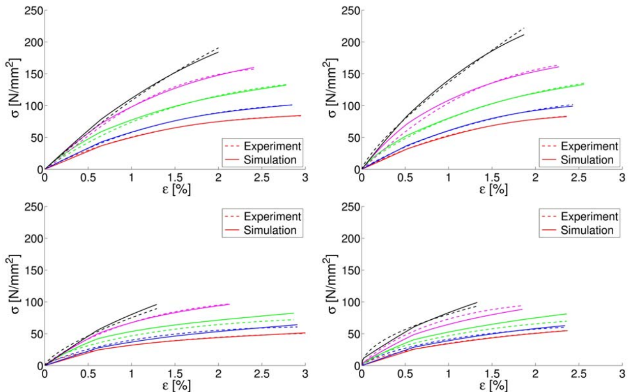
Abb. 7.30: Vergleich gemessener und simulierter Dehnratespektren, PP-LGF 40, Fasern in Zugrichtung (oben), Fasern quer zur Zugrichtung (unten), lokale Auswertung am Versagensort (links), gemittelte Dehnung in Probenmitte (rechts)
