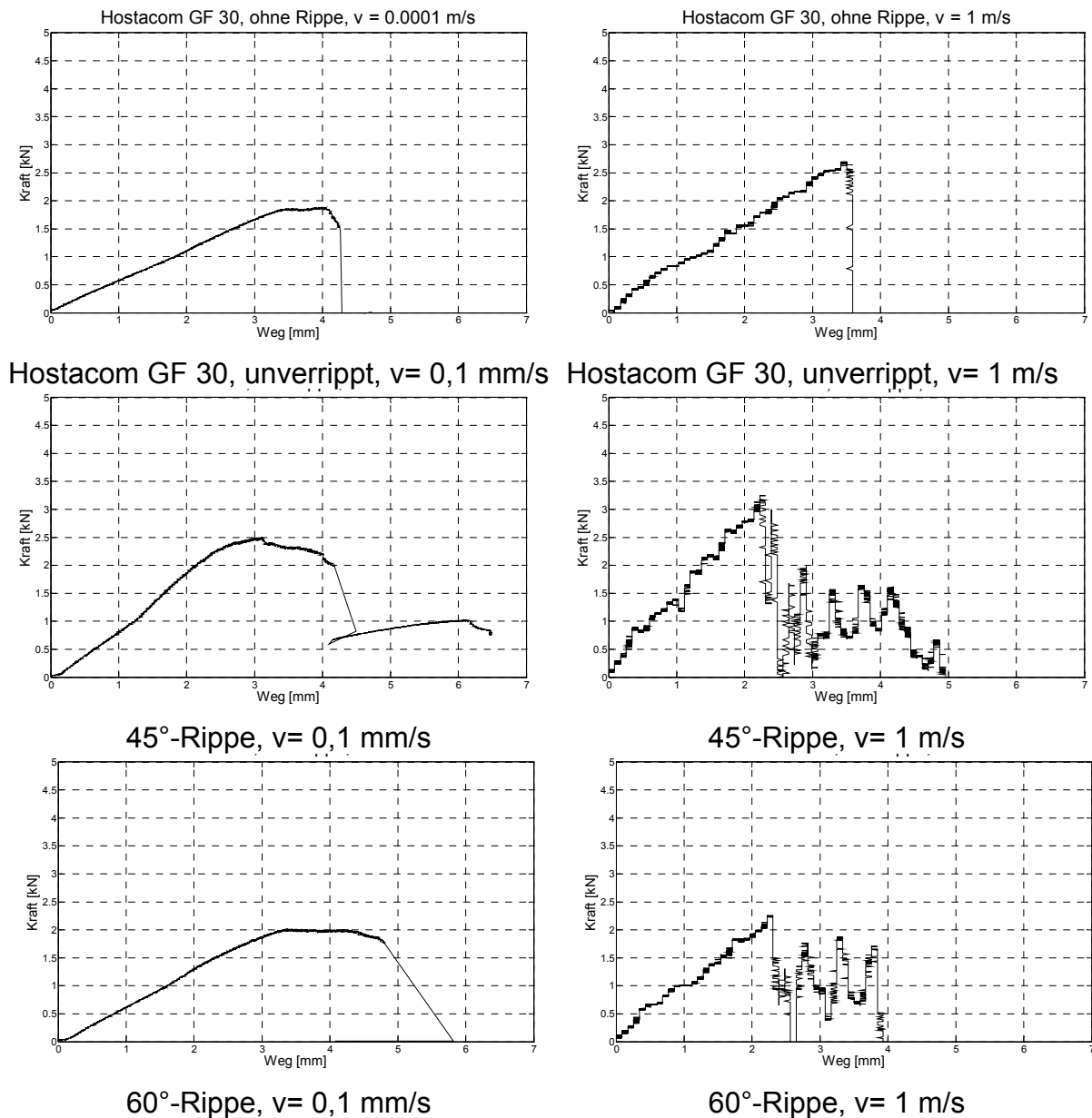
Abb. 5.28: Kraft-Weg-Verlauf, Stirnzugversuch Bauteildemonstrator aus Hostacom PP-GF 30, v_{\text{Abzug}} = 0,1 mm/s und 1 m/s
