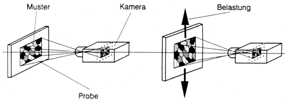
Abb. 4.15: Verfahren der Grauwertkorrelation
