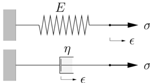
Abb. 2.4: Hooke'sches Federelement und Newton'scher Dämpfer
