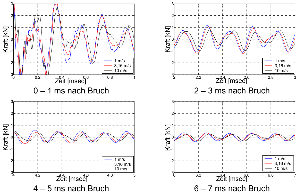
Abb. 6.4: Ausschwingverhalten des Kolbens nach Zugversuchen bei 1 m/s, 3,16 m/s und 10 m/s, Intervalle bis 7 ms nach Bruch
