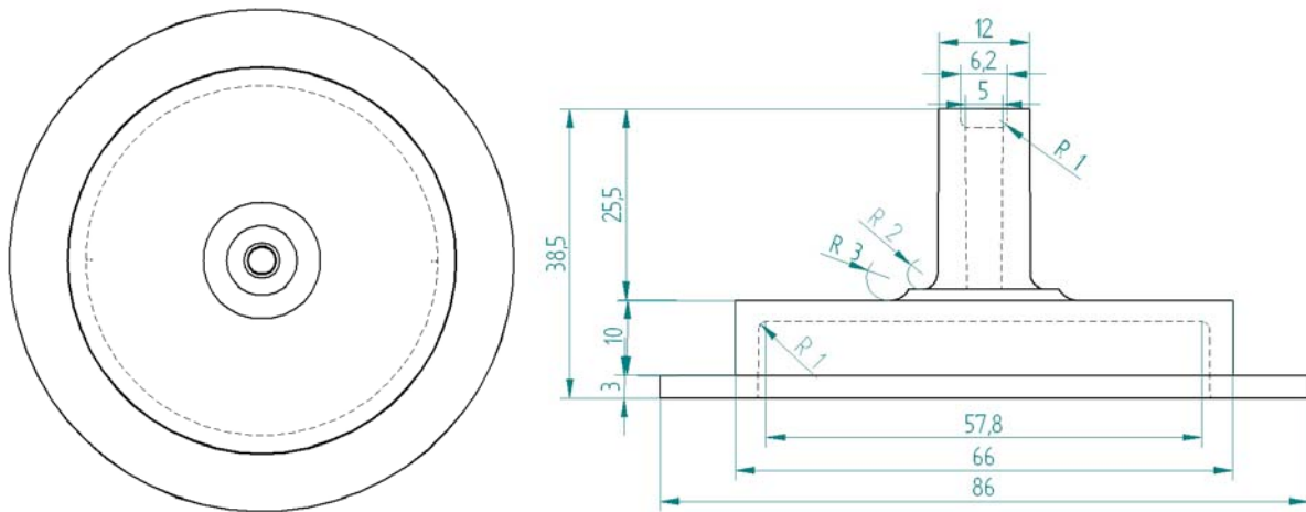
Abb. 3.16: Bauteildemonstrator in unverrippter Ausführung
