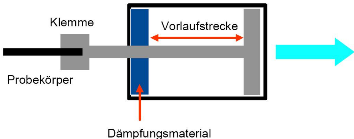
Abb. 4.3: Prinzipskizze Schnellzugversuche [103]
