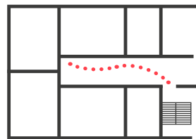
akzeptiertes Risiko: nur ein Rettungsweg mit max. 22,5 m Lauflänge
