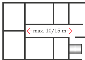
akzeptiertes Risiko: nur ein Rettungsweg
